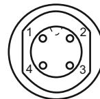
Вид со стороны распайки корпуса с контактами (разъем ключом вверх)
